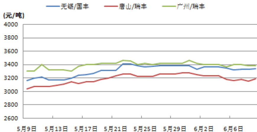
图 1：本周主要城市 2.5mm 热轧带钢价格走势图
