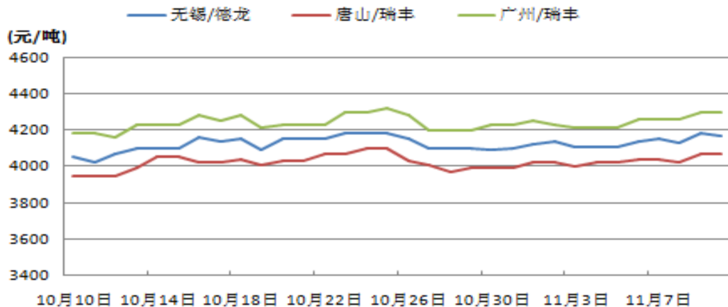
图 1：本周主要城市 2.5mm 热轧带钢价格走势
