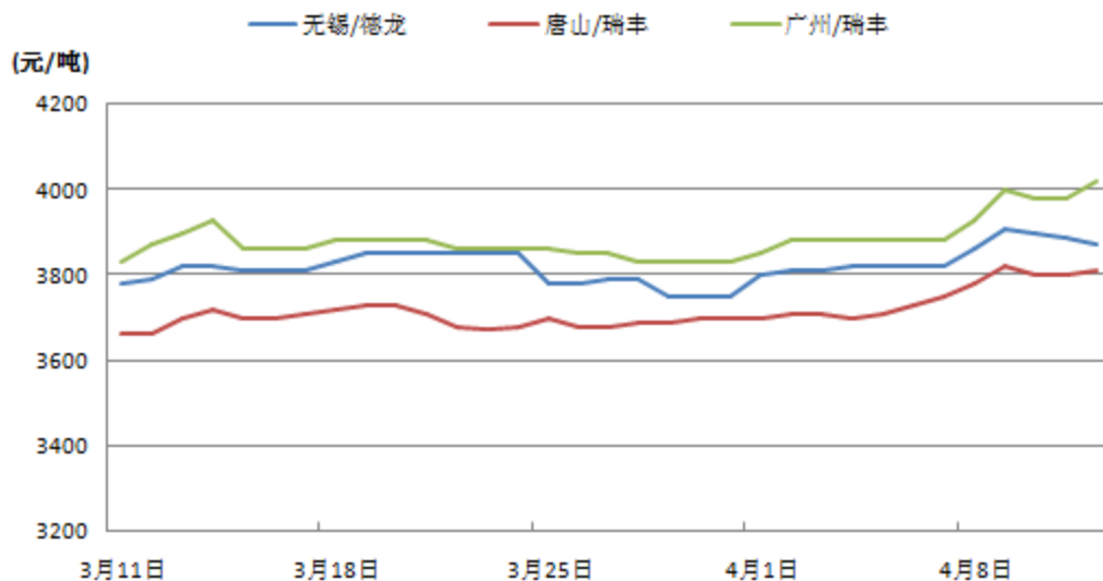
图 1：主要城市 2.5mm 热轧带钢价格走势
